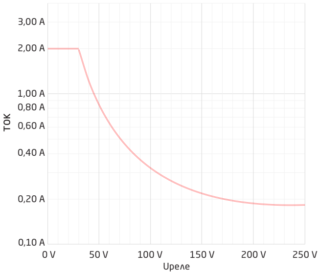
Графическое отображение [1380 \times U_{\text{реле}}^{-2} \times 1,0085 U_{\text{реле}}] :
